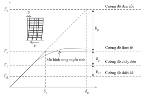
Hình 3. Đường cong quan hệ lực cắt và chuyển vị
