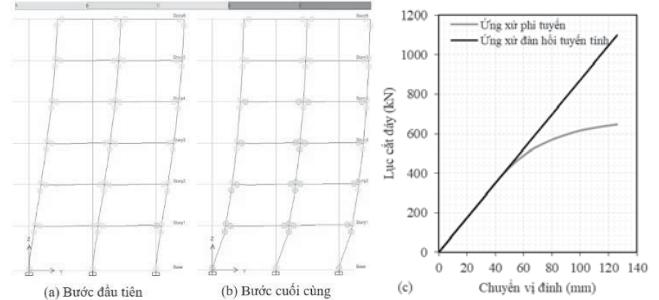
Hình 11. Phản ứng động đất của công trình 6 tầng
